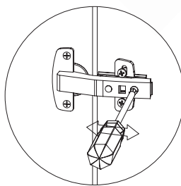
Петля без доводчика
