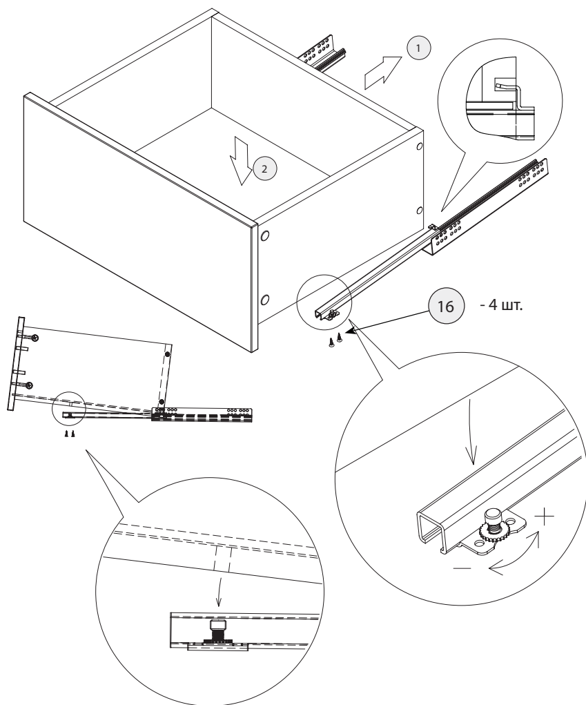
Регулировка ящика по высоте производится с помощью поворота регулировочного колесика (+3 мм)
