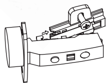
Петля без доводчика
