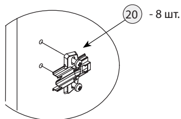
Установка петель на дверь
