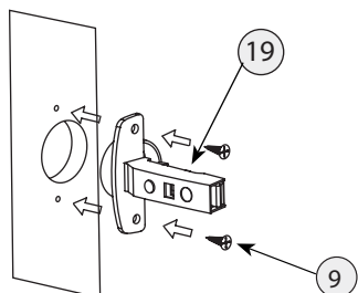
Установка петель на дверь
