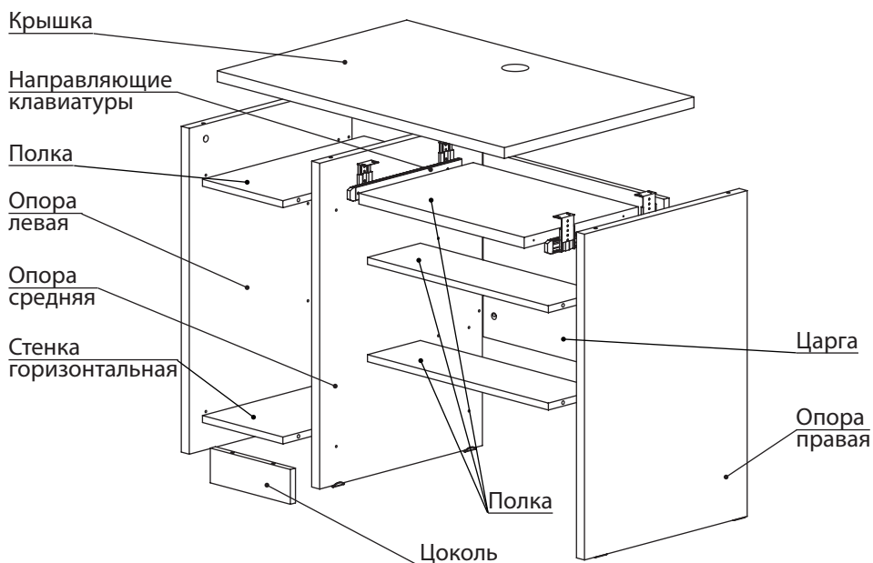
Правое исполнение
